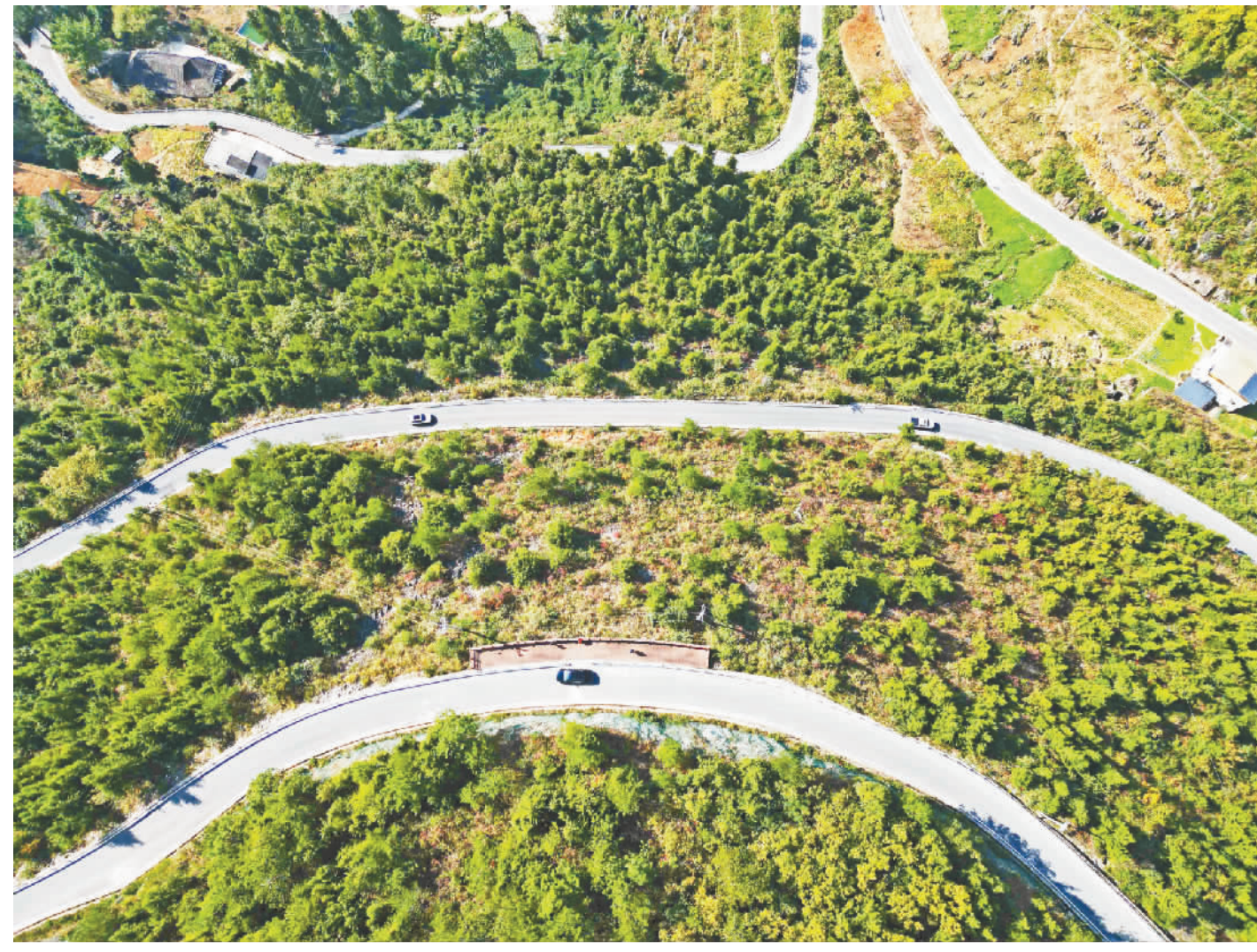
哨路村境内的“四好农村路”。
